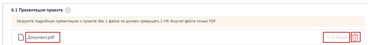
Рисунок 31. Загруженный файл
